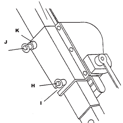
OUTSIDE FACE OF TRIPOD LEG CARA EXTERNA DE LA PATA DEL TRÍPODE FACE EXTÉRIEURE DE LA PATTE DU TRÉPIED
