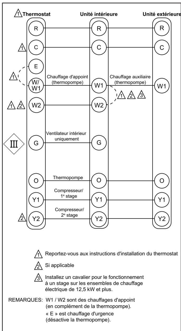
FIGURE 2. Désignation des thermostats non communicants
