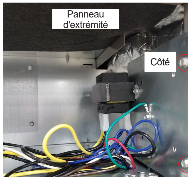
FIGURE 3. Connexions électriques (Configuration ascendante)
