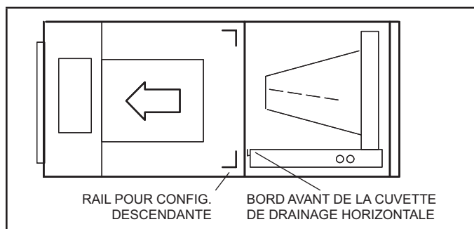
FIGURE 11. Configuration pour refolement du côté gauche
