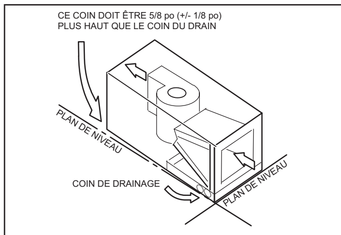
FIGURE 13. Inclinaison de l'unité pour un drainage correct INSTALLATION DU DRAIN DE CONDENSAT
