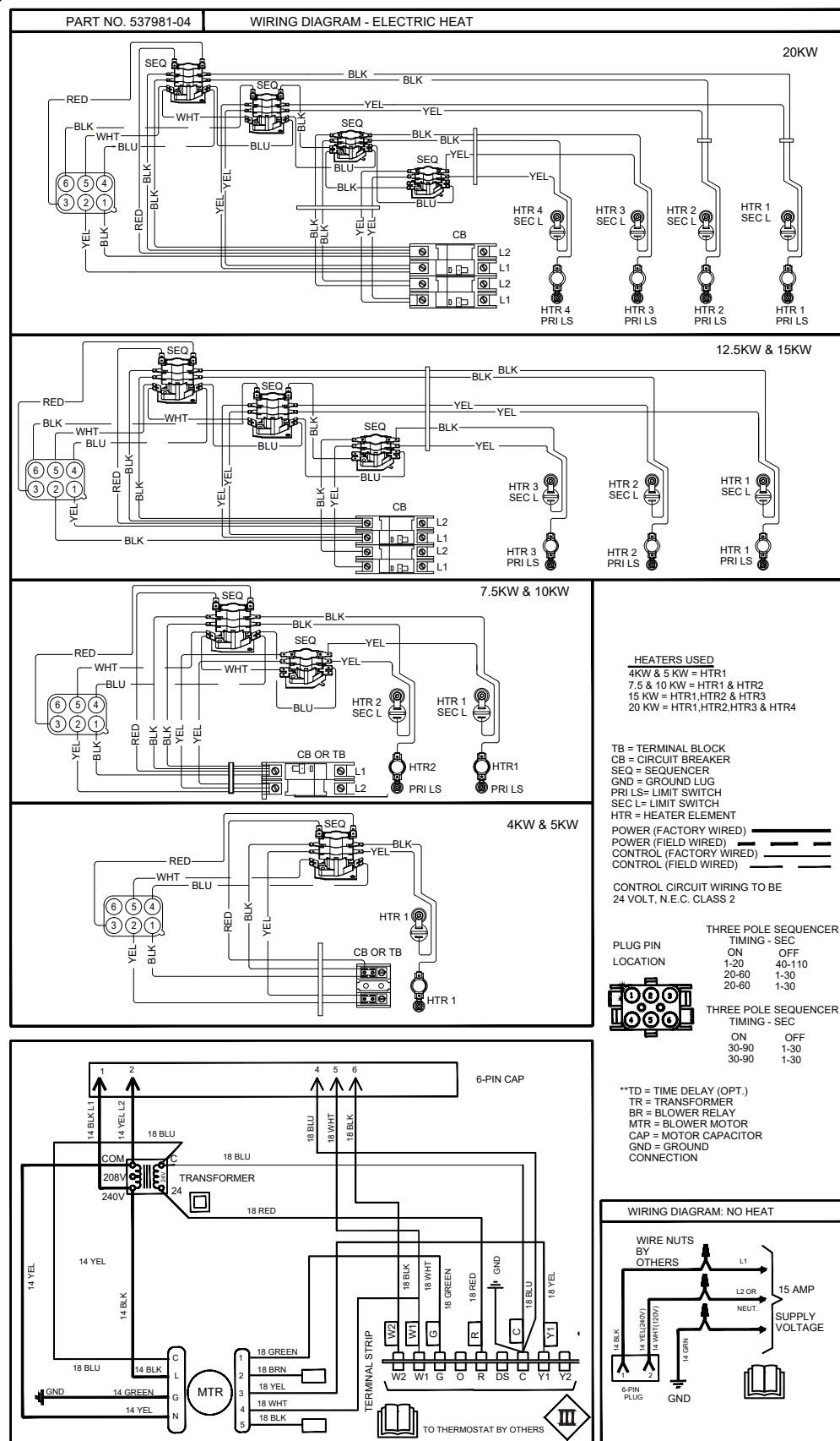
FIGURE 1. Schéma de câblage typique - Ventilo-convecteur CBA25UHE avec chauffage électrique - CT
