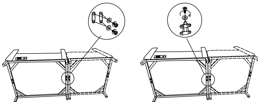
WASHER – QTY: 2
