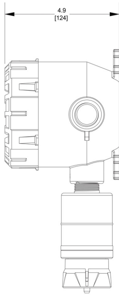
Fig. 48 Deep Lid Depth
