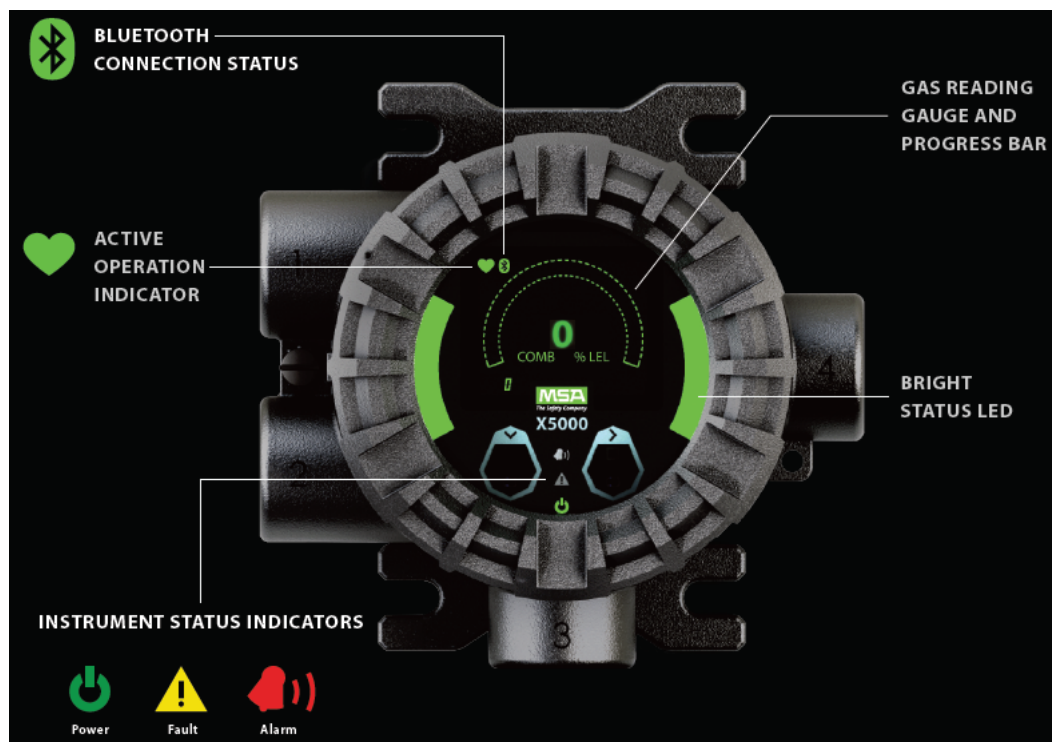
Fig. 1 OLED Display
