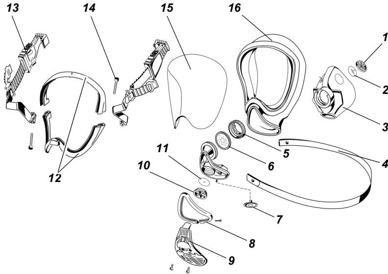
Fig. 3 Vista despiezada de la máscara
