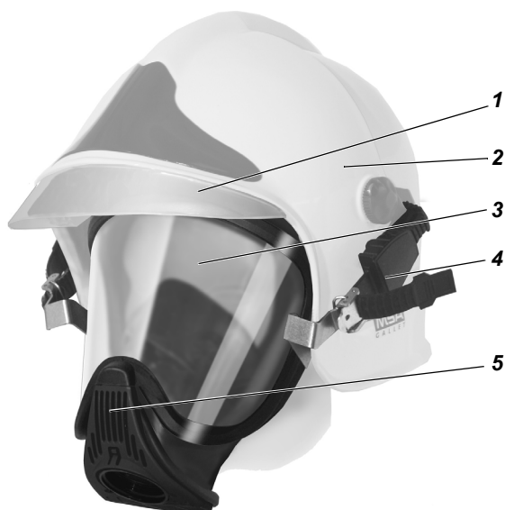
Fig. 1 Vista general de la combinación de máscara/casco
