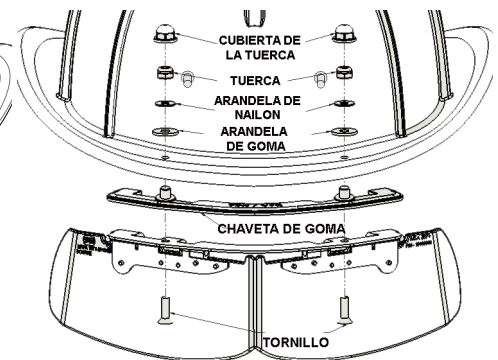
Fig. 6 Montaje de la visera plegable Bourke en los cascos de cuero
