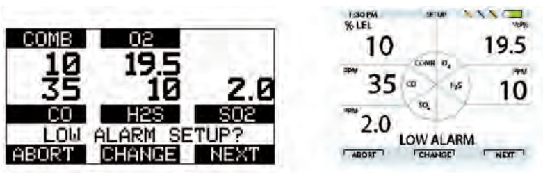
Figura 3-5. Ajuste Valor Alarma de Sensor
