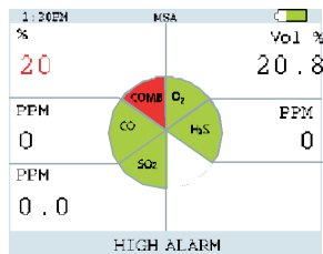
Figure 2-6. Conditions d'alarme (ici Alarme Haute)
