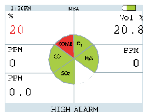
Figura 2-6. Estados de Alarma (en este caso alarma alta)
