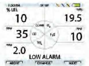
Figure 3-5. Réglage alarme capteur
