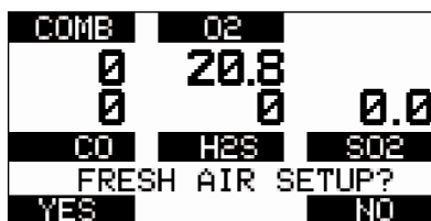
Figure 3-1. Réglage à l'air frais
