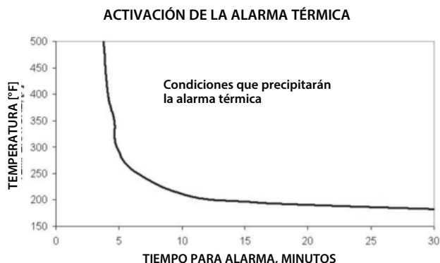
Gráfico 4: Curva de activación de la alarma térmica del módulo de control del FireHawk M7XT
