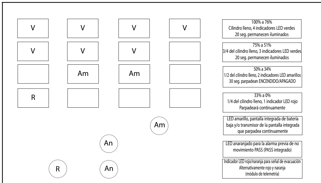
Gráfico 1: Patrones LED de la pantalla integrada del FireHawk M7 para las máscaras de aire FireHawk M7XT
