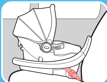
Correa del acoplamiento de anclaje inferior
